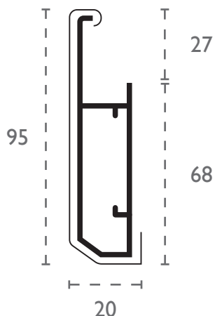
COTAS / MEDIDAS (mm)
