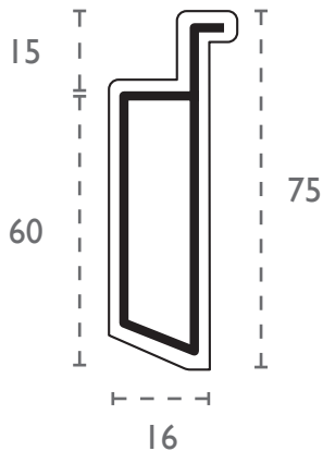
COTAS / MEDIDAS (mm)
