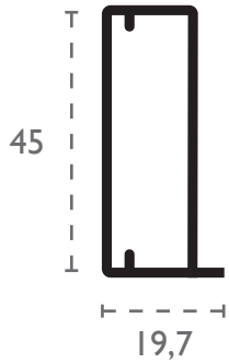
COTAS / MEDIDAS (mm)
